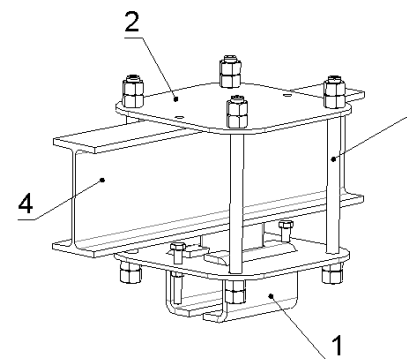
Рисунок 6.1.1- Монтаж универсального кронштейна vрго DL AV01
