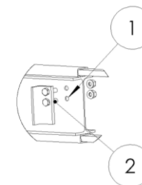
Рисунок 6.7- Монтаж концевого ограничителя vрго DL H02
