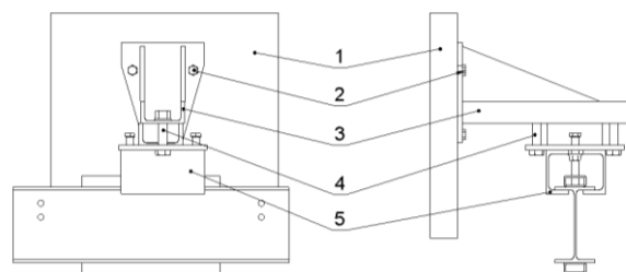
Рисунок 4.5- Крепление при помощи консольного кронштейна vрго DL AV02
