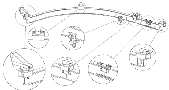
Рисунок 4.1- Общая схема анкерной системы VENTO «ДВУТАВР»
