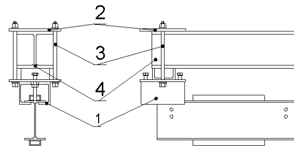
Рисунок 4.2 - Крепление без сверления отверстий в несущей конструкции
