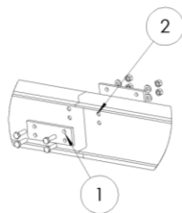
Рисунок 6.4- Монтаж соединительного элемента vрго DL L01
