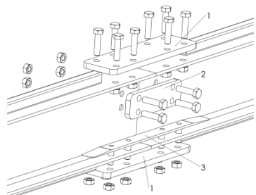
Рисунок 6.2- Монтаж силового соединительного элемента
